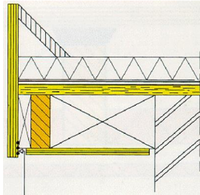
Figuur 7 Voorbeeld uitvoering van een dakoverstek.
