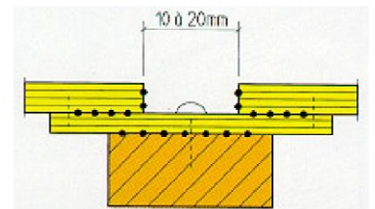
Figuur 4 Verticale naadvariant.
