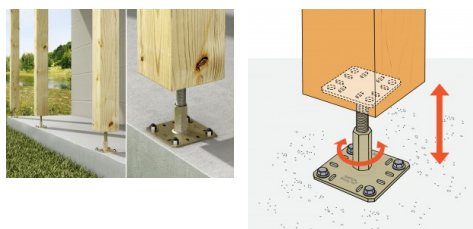
Bevestiging van kolomvoet PPRC op harde ondergrond.
